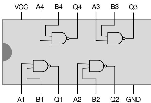
Abbildung 8 74HC00 NAND-Chip
