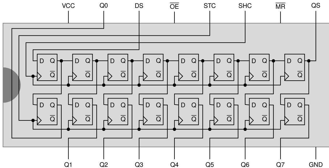
Abbildung 12 74HC595 Schieberegister
