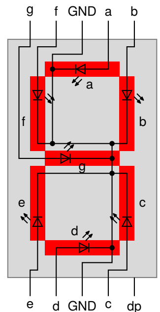
Abbildung 6 Schaltung der Segmentanzeige
