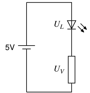
Abbildung 3 Leuchtdiode mit Vorwiderstand
